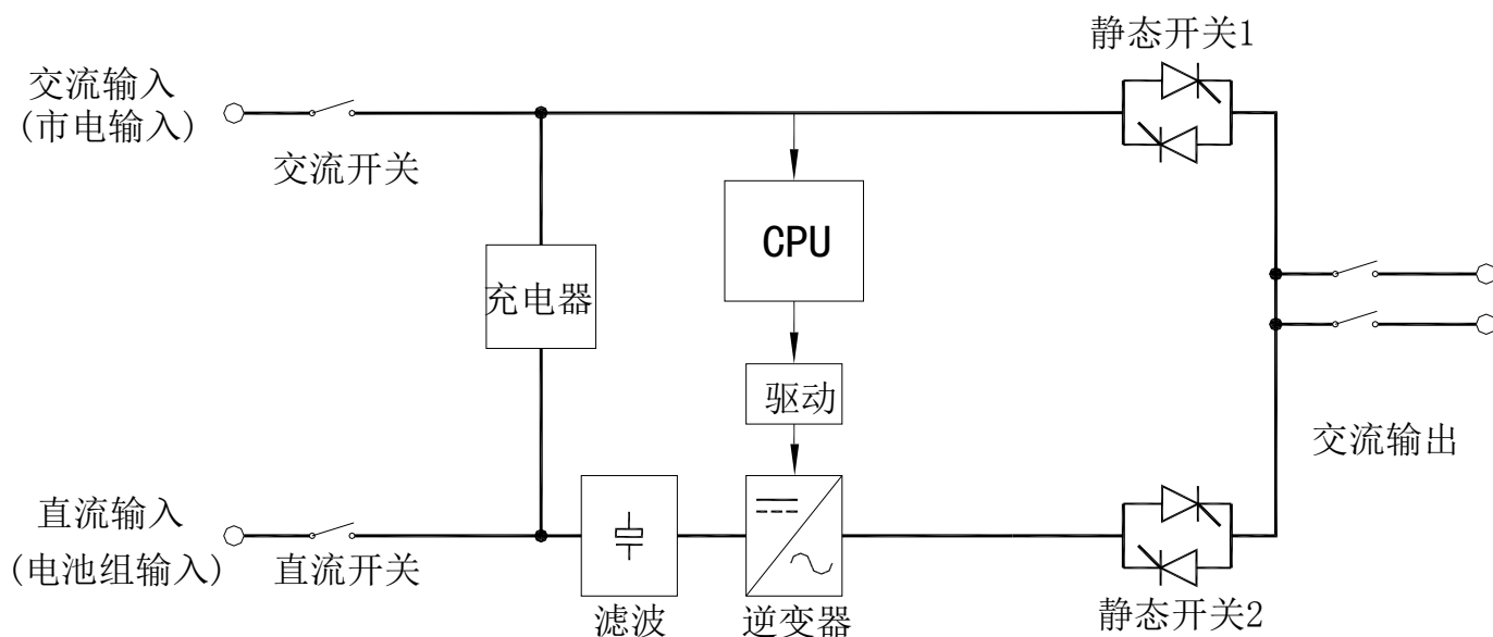
原理框图
