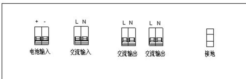
输入输出接线
